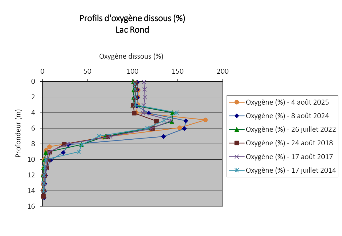
Figure 4: Profils d'oxygène dissous au lac Rond
