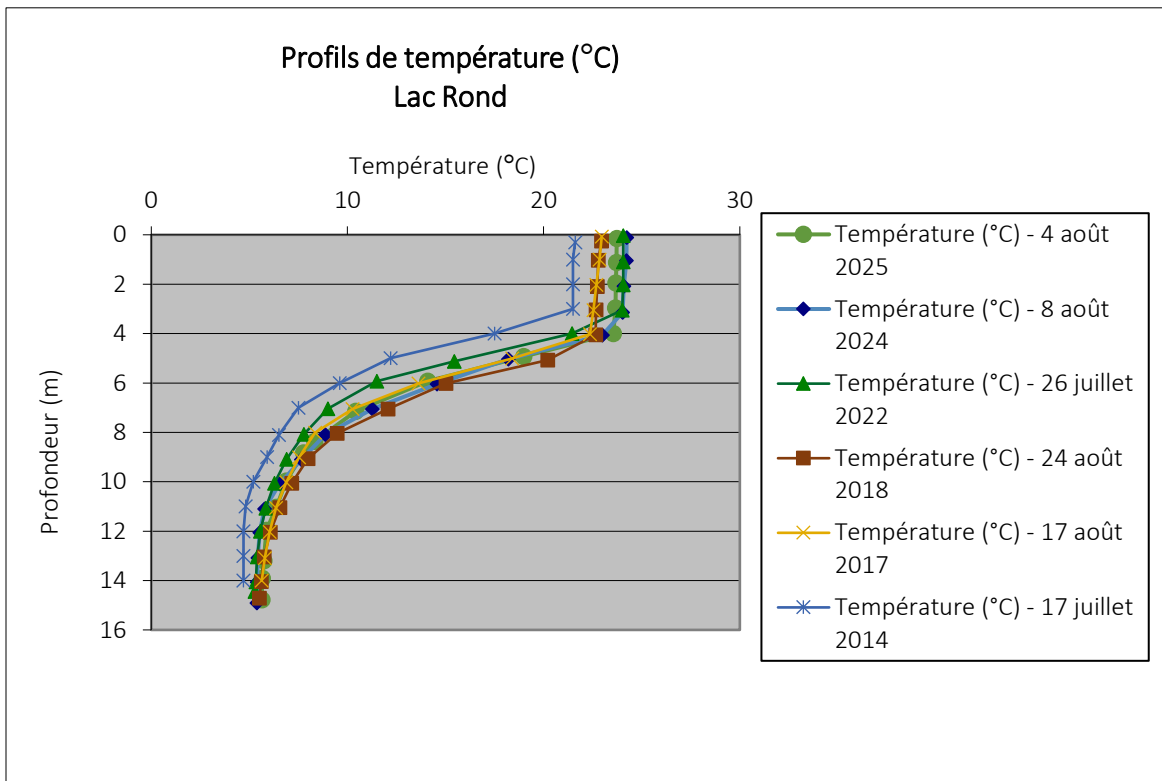
Figure 3: Profils de température au lac Rond
